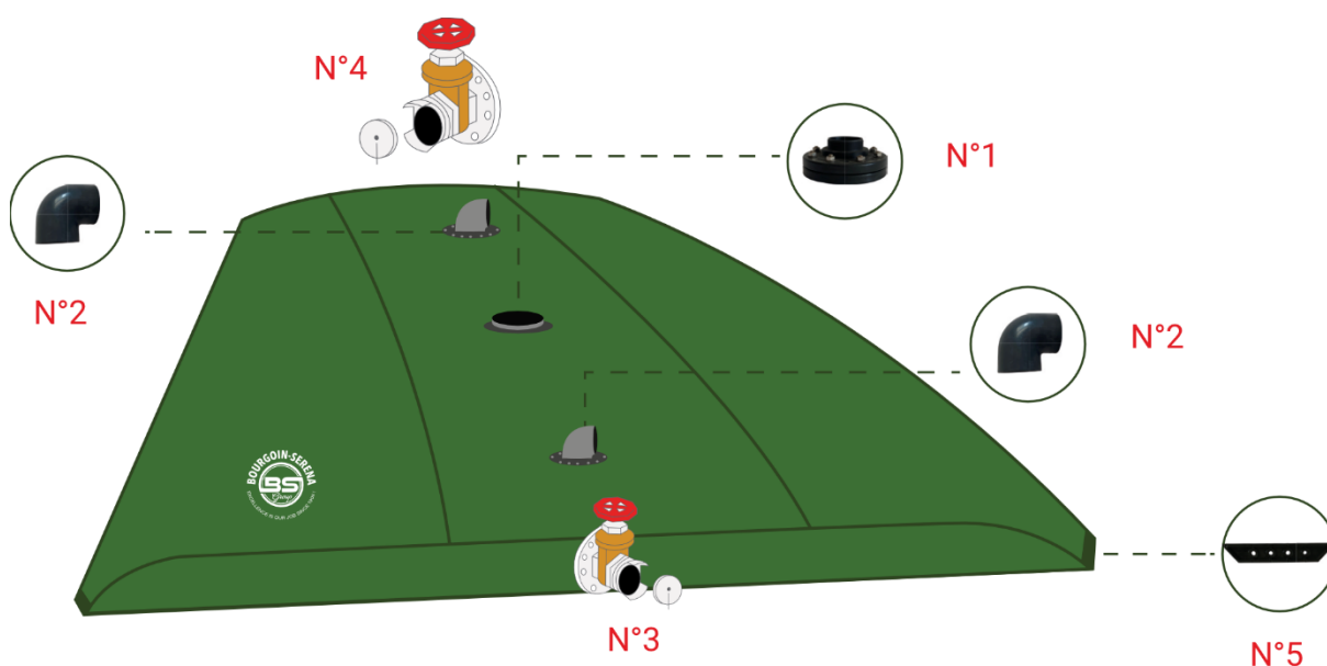
Obr. 1: Schematický nákres flexibilní nádrže
