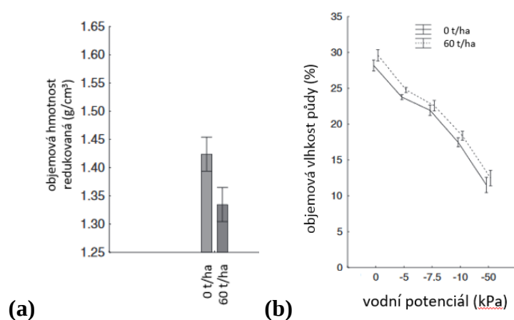
Obr. 13: Změny v objemové hmotnosti redukované půdy (a) a dostupnost vody (b) při přidavku biouhlu 60 t/ha.
