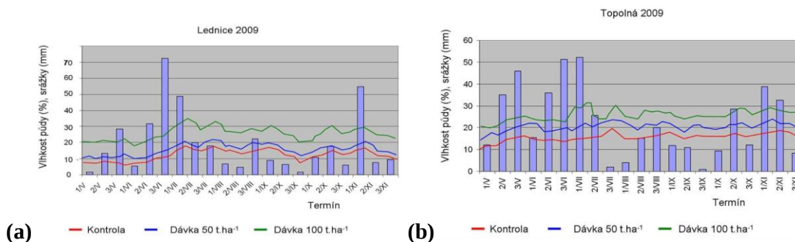
Obr. 9: Aplikace kompostů výrazně zvyšuje hodnoty objemové vlhkosti půdy díky zvýšení její vododržnosti, a to až o několik desítek procent (výsledky pokusu s aplikací kompostu v písčité půdě černozevního typu na dvou stanovištích: v obou případech došlo k výraznému zvýšení vododržnosti a eliminaci rizika poklesu obsahu vody pod mez její dostupnosti).
