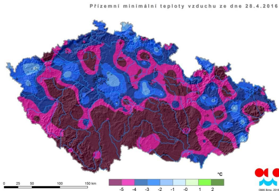
Obr. 1 Přizemní minimální teplota vzduchu ze dne 25. 4. 2016 na území České republiky (Zahradníček et al., 2017)
