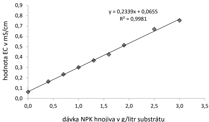
Obr. 1: Závislost hodnot specifické elektrické vodivosti (EC v mS/cm), stanovených dle ČSN EN 13038, u lesnického substrátu s podílem tmavé rašeliny na dávkách základního hnojení plným hnojivem PG Mix (v g hnojiva/litr substrátu); orig. in Šrámek a Dubský (2014)
